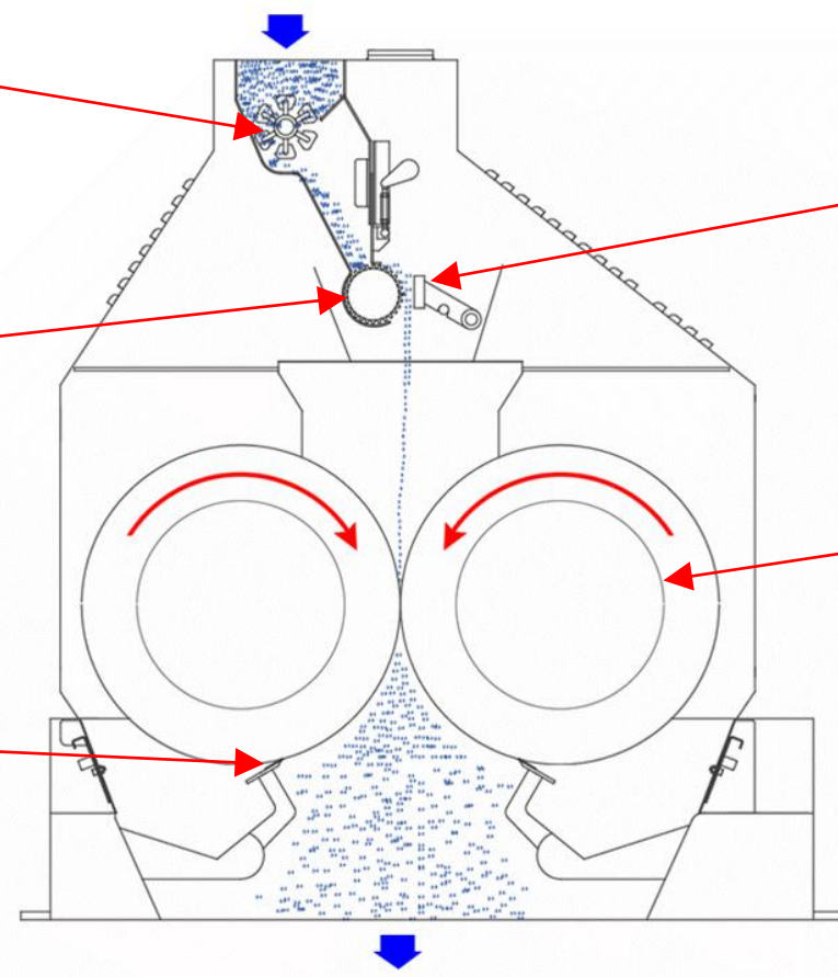
均料装置 Distributor
